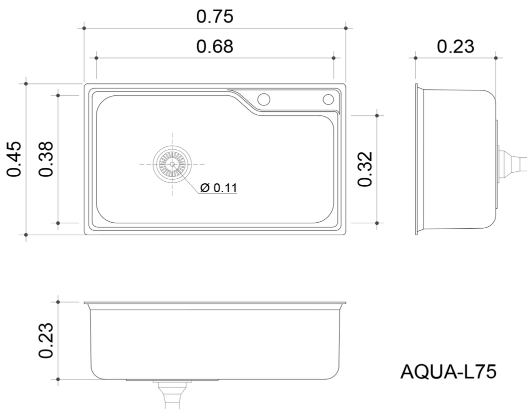
COLADOR PARA AQUA L-75
